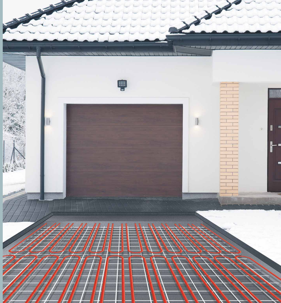
Вариант установки нагревательного кабеля для обогрева подъездных путей
